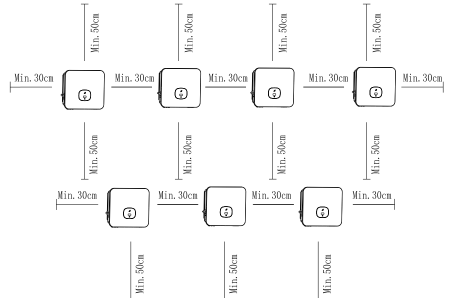
Fig 5.3 Dimensões de instalação de múltiplos inversores
