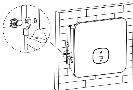
Fig 6.1 Diagrama de aterramento
