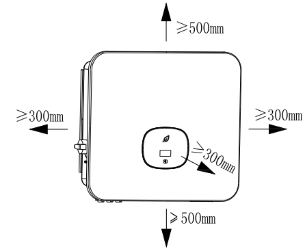
Fig 5.2 Dimensões de instalação de 1 inversor
