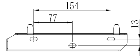
Fig 5.7 Especificações de montagem na parede
