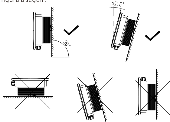
Fig 5.1 Diagrama de instalação
