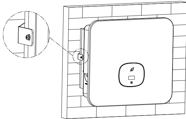
Fig 5.9 Diagrama esquemático de instalação do inversor na parede
