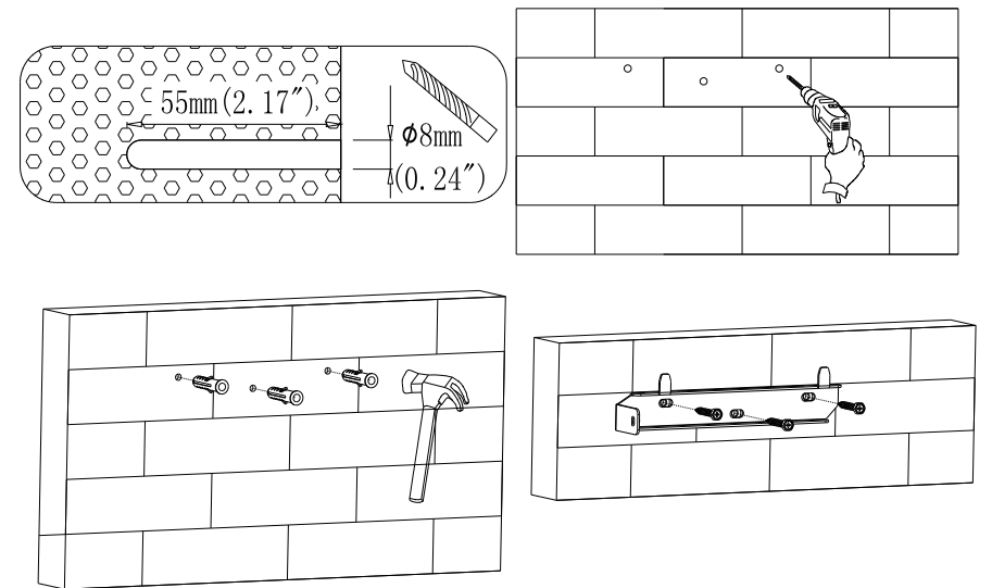
Fig 5.8 Diagrama esquemático de instalação do suporte de parede
